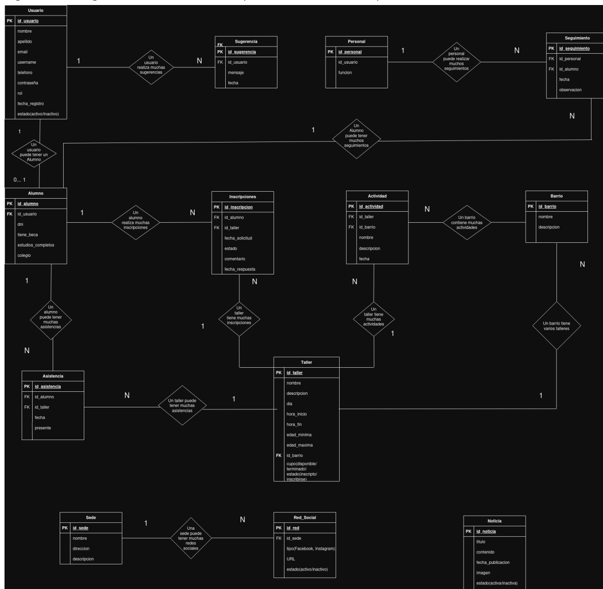
Figura 1 - Diagrama entidad-relación(realizado en draw.io).
